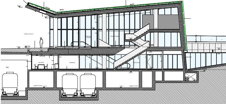
coupe longitudinale
