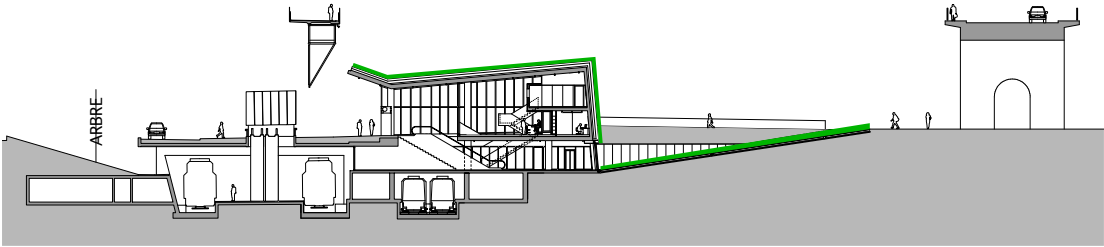
coupe longitudinale
